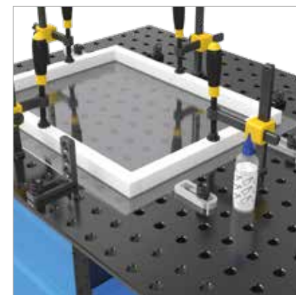
Ragasztott műanyag profilok
